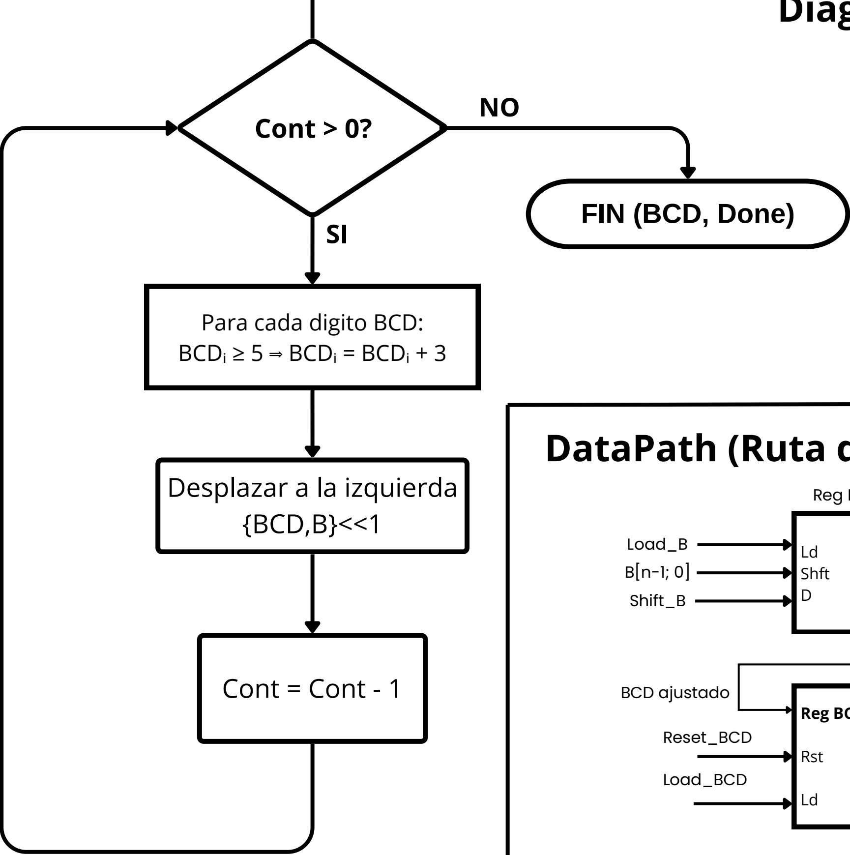
Diagrama de flujo Double Dabble
