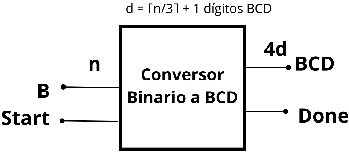
Diagrama de caja negra Double Dabble
